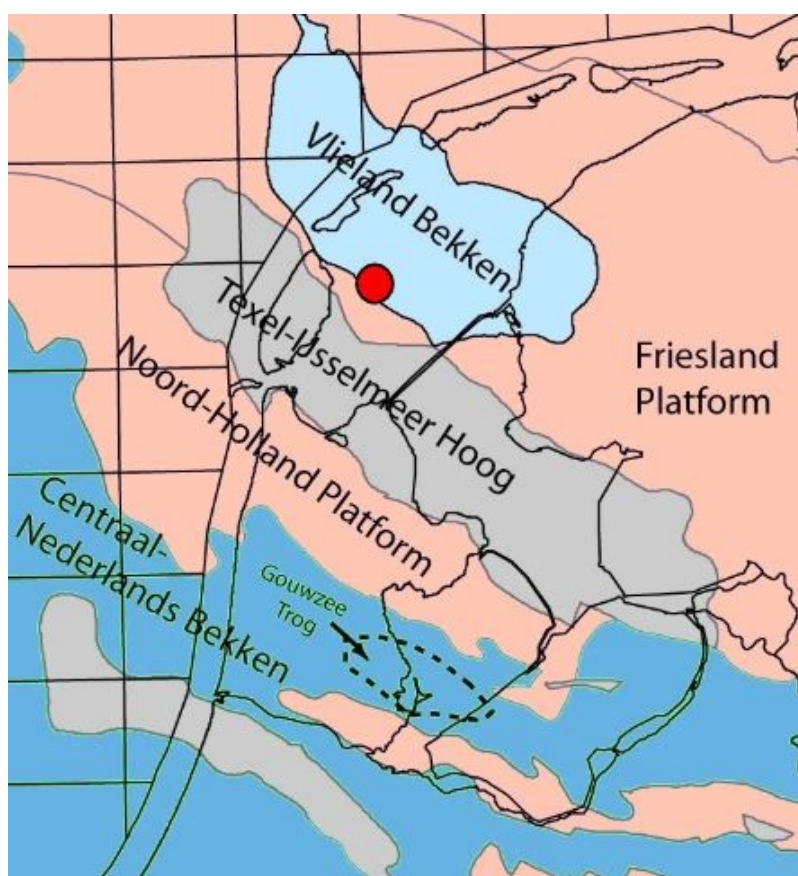
Figuur 2: Geografische ligging van de Gouwzee Trog.
